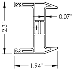
11 ASTRAGAL
